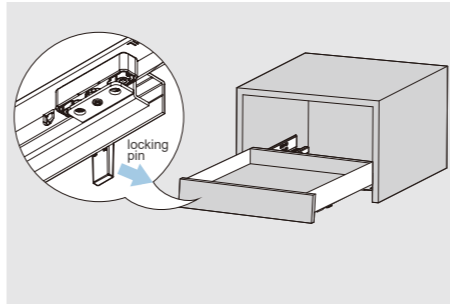
снимите направляющие с замка
